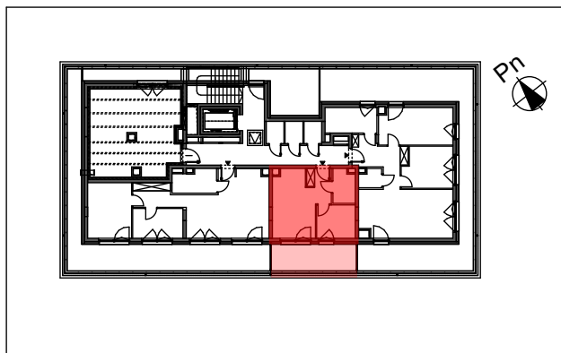
SCHEMAT OSTATNIEGO PIĘTRA BUDYNKU 2
