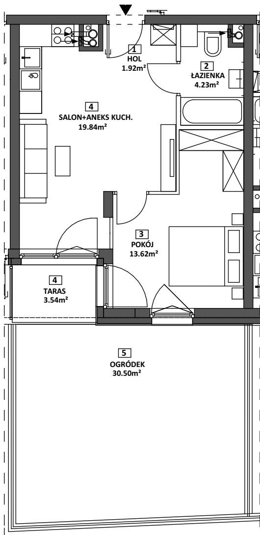
SCHEMAT PARTERU BUDYNKU 4
